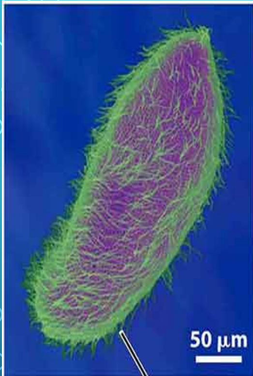
Cilia
