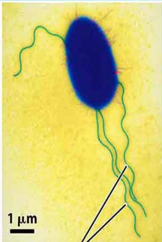
Flagella
